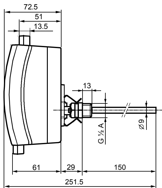
Контроллер с защитной гильзой
